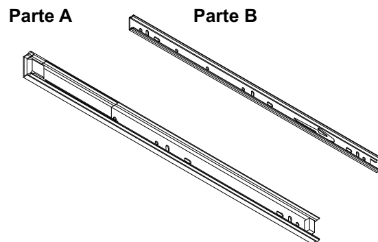
Passo 02 Com as partes da corrediça separadas, fixar-las no móvel.
