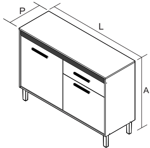
BALC 2PT1G-120 PRODUTO MONTADO: A: 870 L: 1200 P: 413 MM
