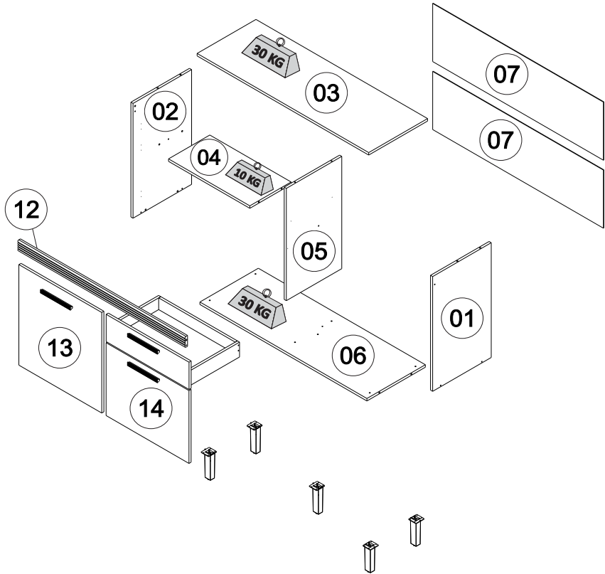
BALC 2PT1G-120 PRODUTO MONTADO: A: 870 L: 1200 P: 413 MM
