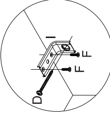
detalhe 08
