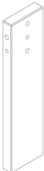
05 Pé Esquerdo Peseira (348 x 90 x 25mm)
