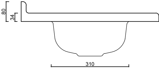
04 Vista lateral
