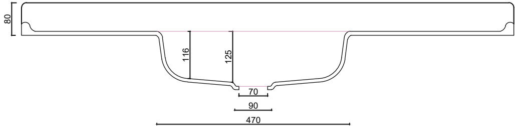
02 Corte AA
