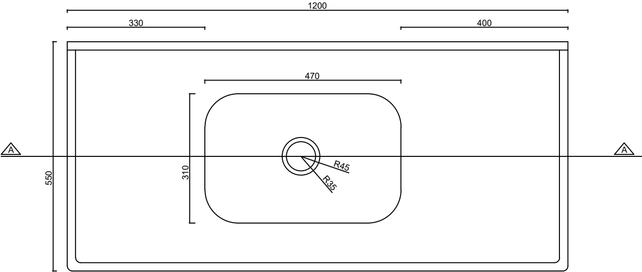
01 Vista Superior
