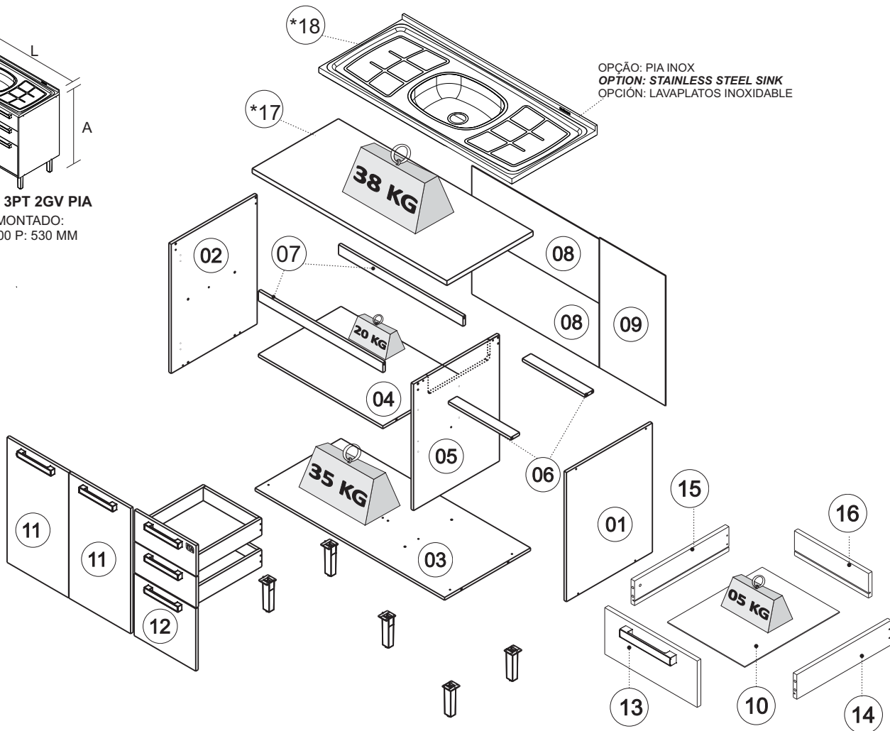
BALC- 120 3PT 2GV PRODUTO MONTADO: A: 876 L: 1200 P: 530 MM
