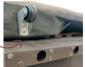
POSICIONE O RODÍZIO COM A RODA PARA O LADO EXTERNO DO SOFÁ. ENCAIXE OS DOIS PARAFUSOS NA POSIÇÃO CORRETA.
