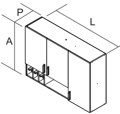
ARM-120 PD 3P-120 GAR PRODUTO MONTADO: A: 800 L: 1200 P: 310 MM
