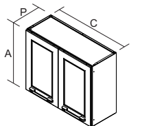
ARM 70 2PT Produto Montado C:700 A:550 P:280 MM
