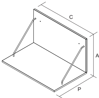
NICHO MICROONDAS 70 Produto Montado C: 690 A: 400 P:430 MM
