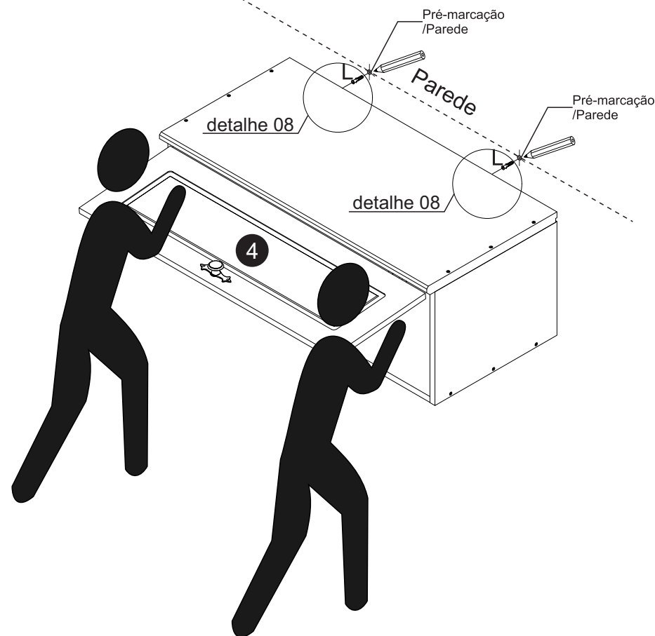
detalhe 08
