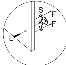
detalhe 14
