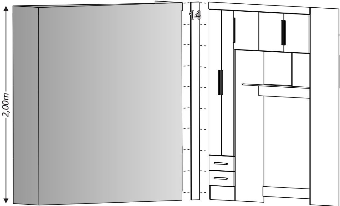
VISÃO FRONTAL FRONT VIEW VISTA FRONTAL
