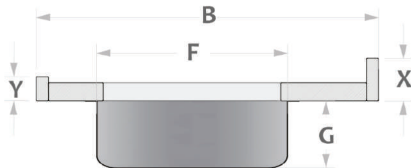
CORTE TRANSVERSAL
