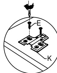
Detalhe 5 detail 5 / detalle 5
