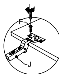
Detalhe 4 detail 4 / detalle 4
