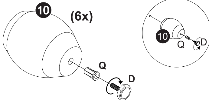
D- Sapata Reguladora 1/4" (6x)
