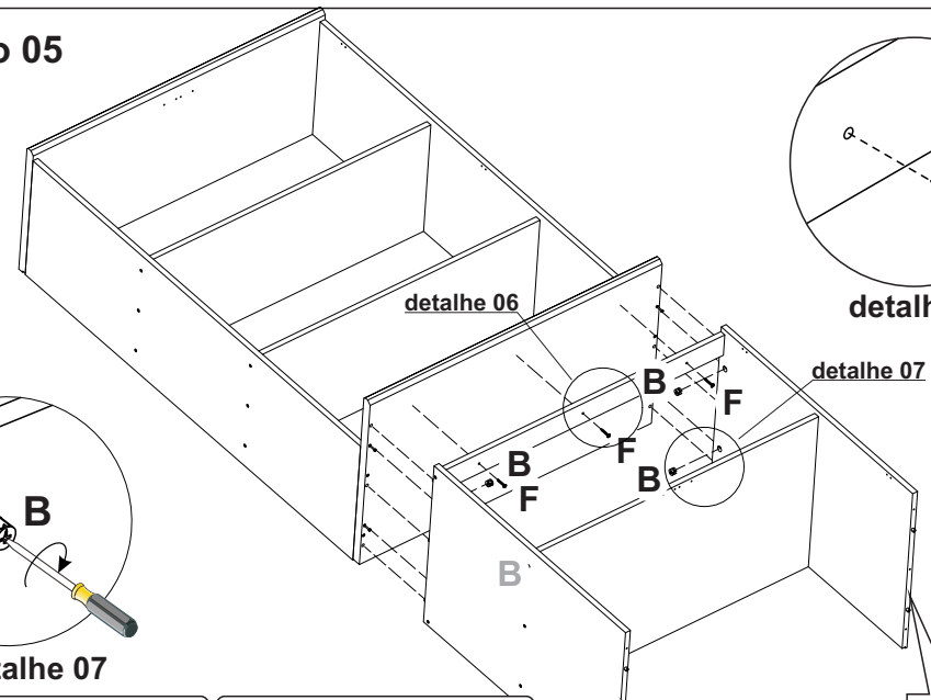
B- Tambor Mini-Fix (4x)
