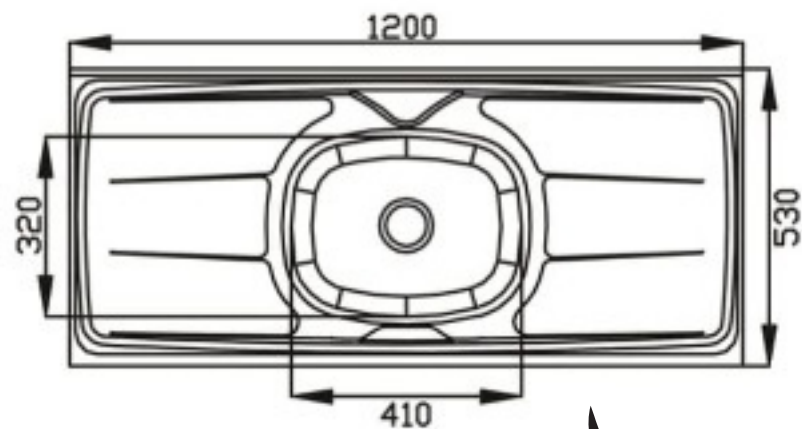
OPÇÃO 02: Para tampo de Inox (Pia)
