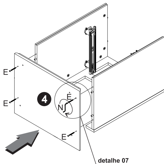
detalhe 07
