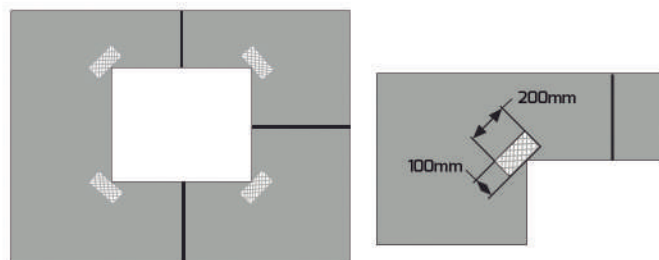
Detalhe de reforço interno de canto para corte tipo "L".
