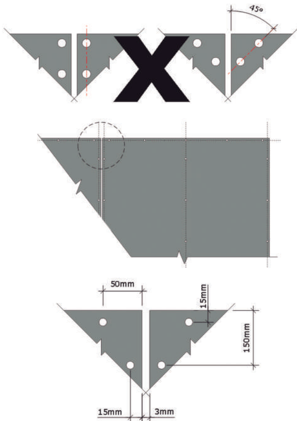
Detalhe das fixações de canto.
