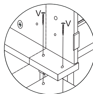
Detalhe 6
