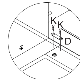
Detalhe 14
