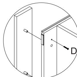
Detalhe 12
