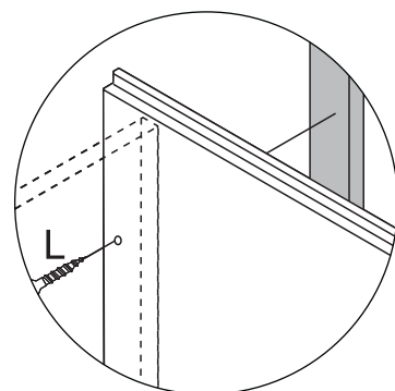
Detalhe 6
