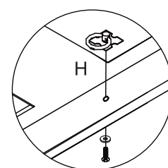
Detalhe 9
