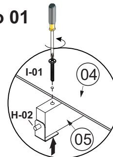
detalhe 04
