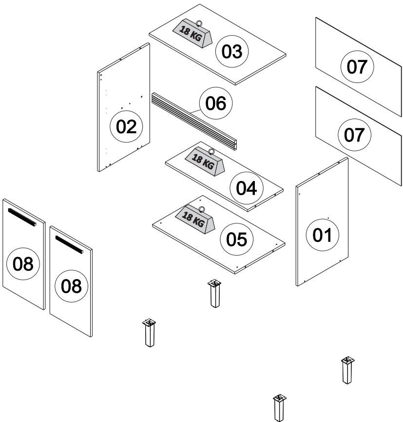
BALC 2PT-70 PRODUTO MONTADO: A: 870 L: 700 P: 413 MM
