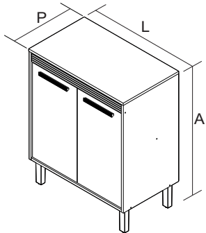
BALC 2PT-70 PRODUTO MONTADO: A: 870 L: 700 P: 413 MM
