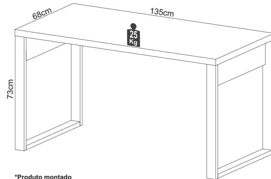
*Produto montado
