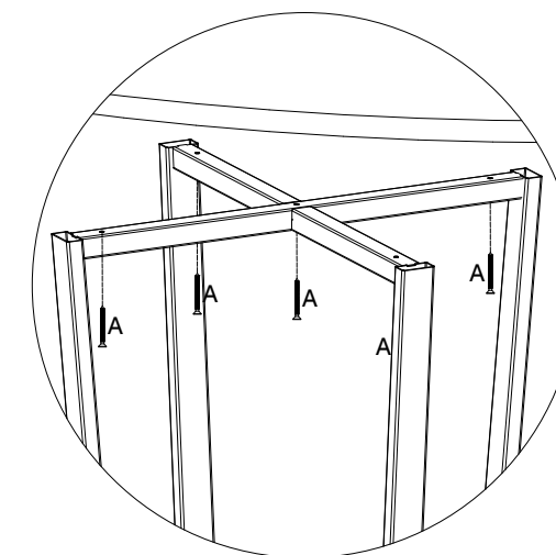
Detalhe 2
