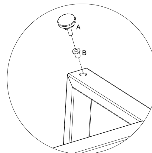
Detalhe 1
