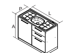
BALC-120 1PT3G PIA PRODUTO MONTADO: A: 900 L: 1200 P: 530 MM
