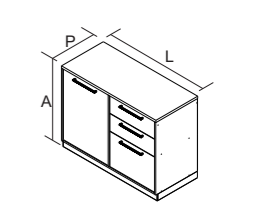
BALC-120 1PT3G PIA PRODUTO MONTADO: A: 900 L: 1200 P: 530 MM
