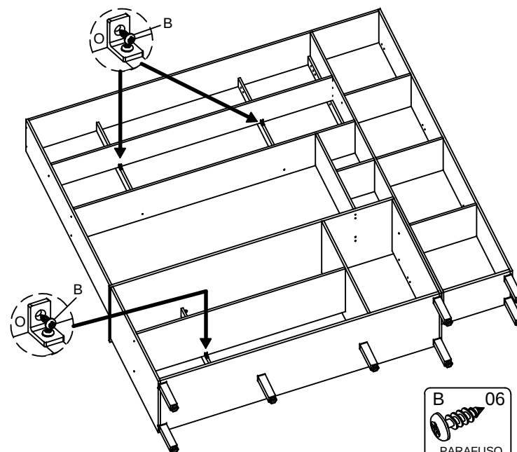
④ FIXAÇÃO DA ESTRUTURA SUP. C/ INF. UPPER STRUCTURE ATTACHMENT INTO LOWER. FIJACIÓN DE LA ESTRUCTURA SUP CON LA INF.
