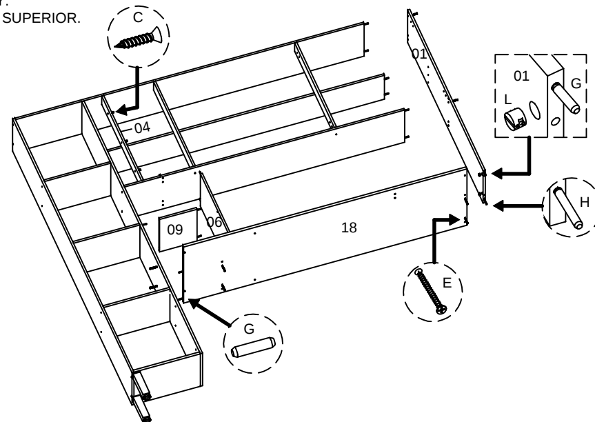
④ FIXAÇÃO DA ESTRUTURA SUP. C/ INF. UPPER STRUCTURE ATTACHMENT INTO LOWER. FIJACIÓN DE LA ESTRUCTURA SUP CON LA INF.
