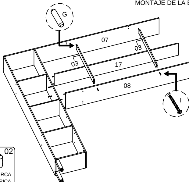
③ MONTAGEM DA ESTRUTURA SUPERIOR. UPPER STRUCTURE ASSEMBLY. MONTAJE DE LA ESTRUCTURA SUPERIOR.
