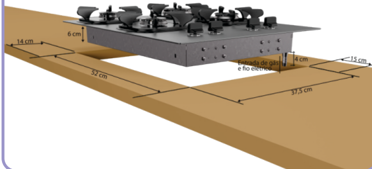
Dimensões do Nicho para modelos de 4 bocas
