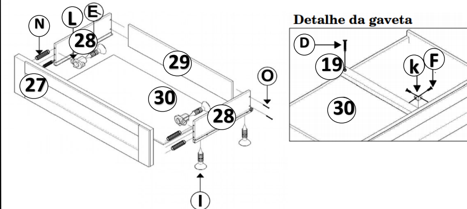
DETALHE 4
