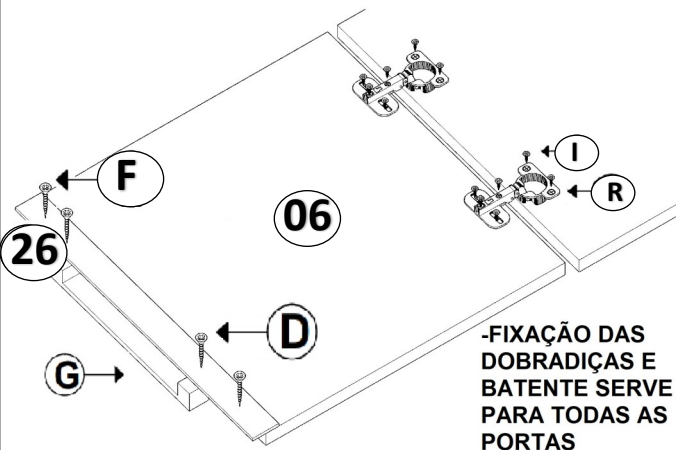
DETALHE 01
