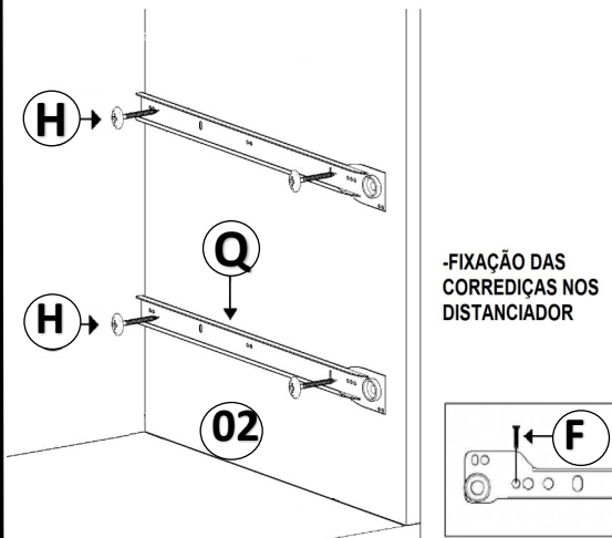
DETALHE 02
