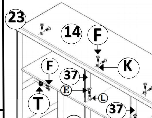
DETALHE 07
