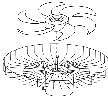
Insira a hélice no eixo do motor alinhando a abertura para encaixar no pino trava
