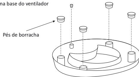
Base do ventilador
