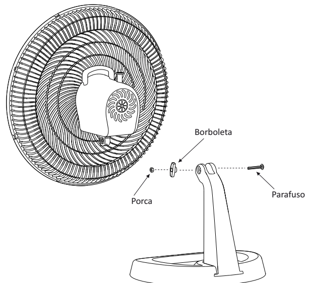
Coloque o motor do ventilador na coluna e fixe com parafuso, porca e a borboleta;
