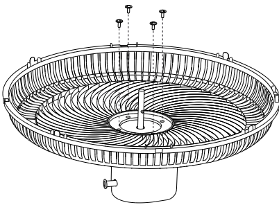
Posicione a grade no motor e aperte com 4 parafusos.
