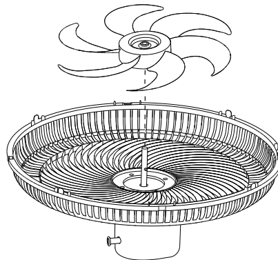
Insira a hélice no eixo do motor alinhando a abertura para encaixar no pino trava
