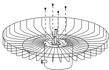
Posicione a grade no motor e aperte com 4 parafusos de 4mm X 12mm.
