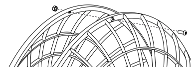
Para ventiladores de 50cm grades plásticas: Alinhe as grades e fixe com parafusos 4mm X 20mm e porcas de 4mm
