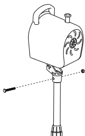
5 - Coloque o ventilador no pedestal e fixe com parafuso 6,35mm (1/4" X 1/2") e porca 6,35mm (1/4" X 7/16").
