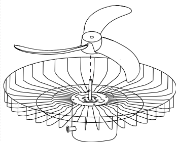
Insira a hélice no eixo do motor alinhando a abertura para encaixar no pino trava
