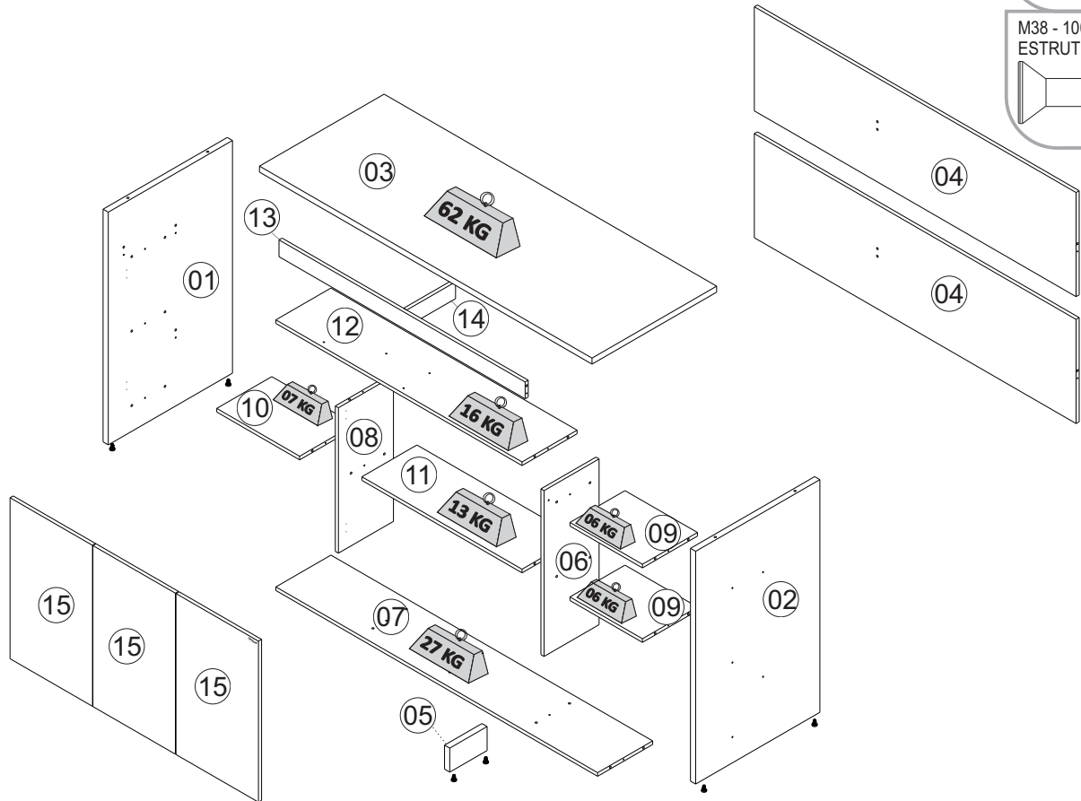
ILHA 2PT GOURMET PRODUTO MONTADO: A: 1010 L: 1600 P: 600 MM
