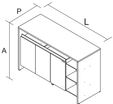
ILHA 2PT GOURMET PRODUTO MONTADO: A: 1010 L: 1600 P: 600 MM
