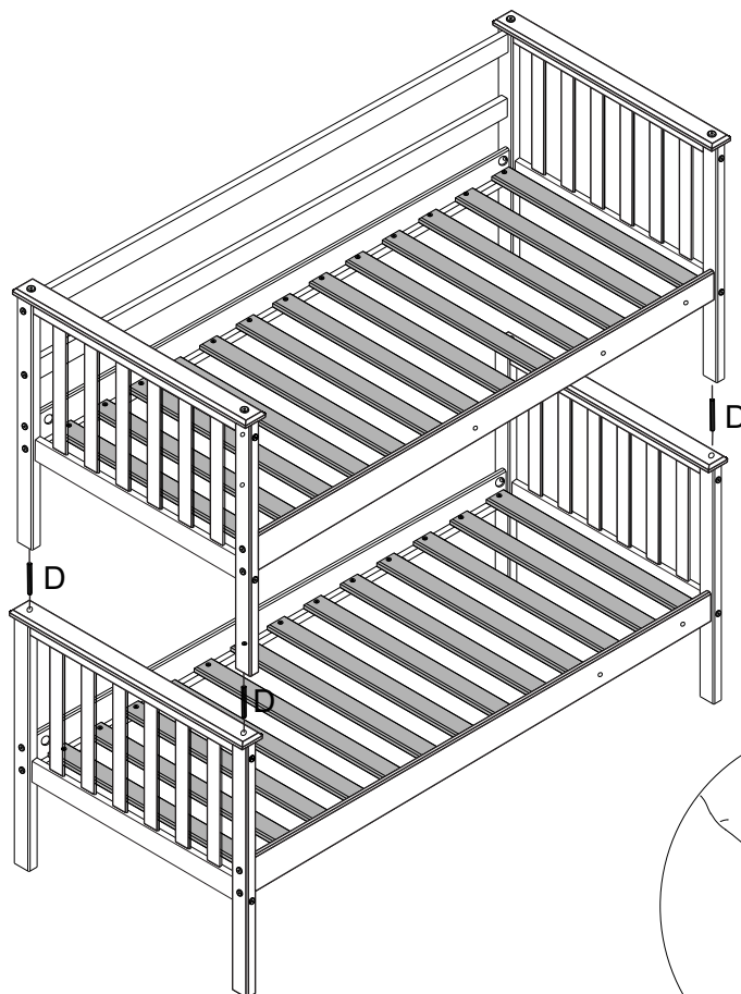
Detalhe 7
