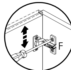
Regulagem Vertical Vertical Adjustment Ajuste Vertical
