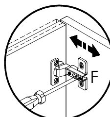
Regulagem Profundidade Depth Adjustment Ajuste Profundidad
