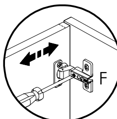
Regulagem Horizontal Horizontal Adjustment Ajuste Horizontal
