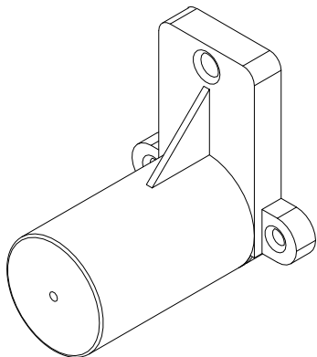
BB- Distanciador de Corrediça T48mm (12x) Cod 2684
