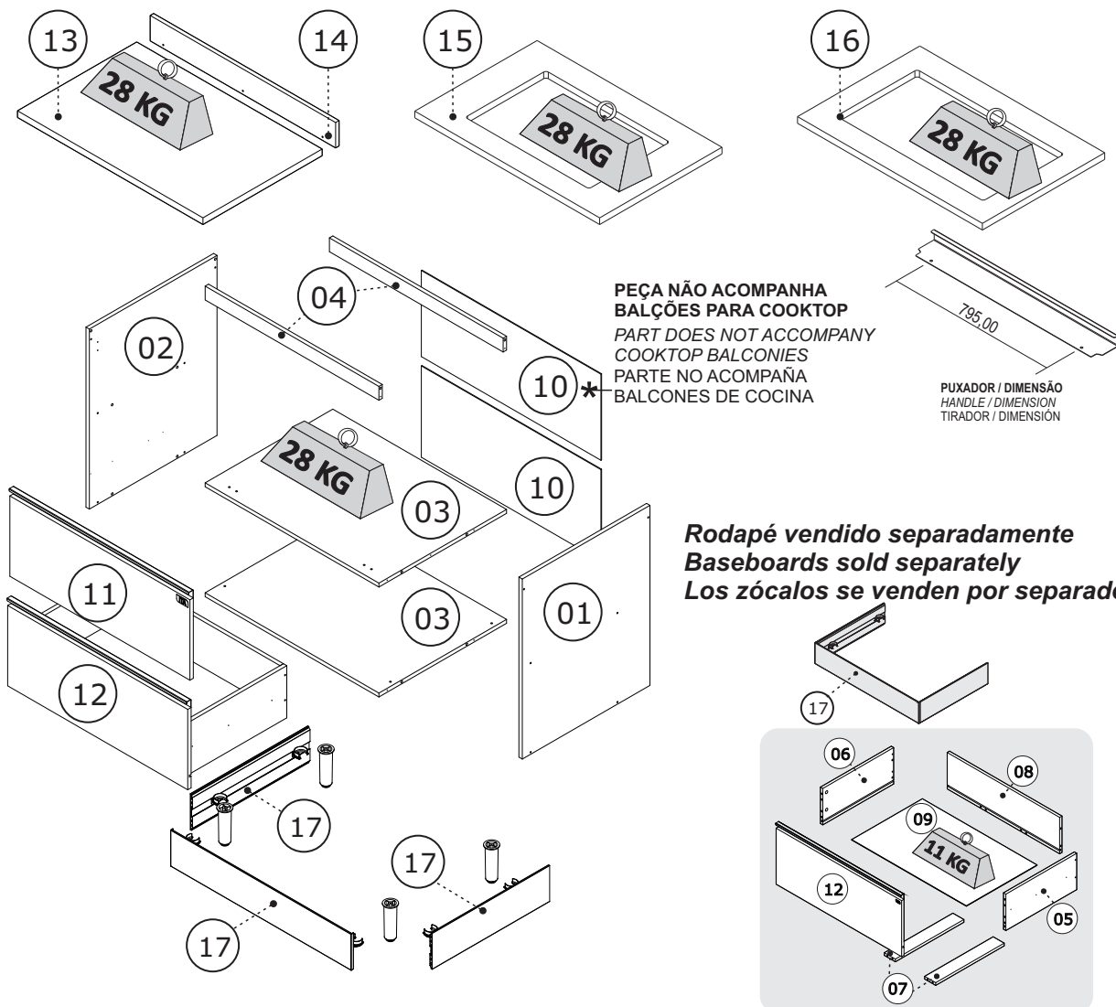
BALC 1PH1G-80 PRODUTO MONTADO: A: 925 L: 800 P: 530 MM
