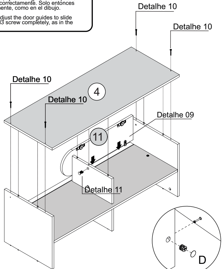
Detalhe 11 Detail/Detalle
