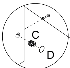
Detalhe 11 Detail/Detalle
