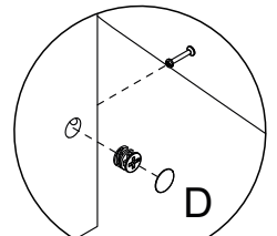
Detalhe 11 Detail/Detalle
