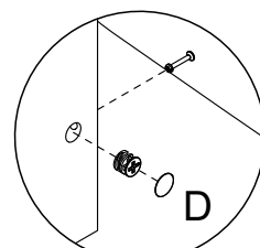
Detalhe 11 Detail/Detalle
