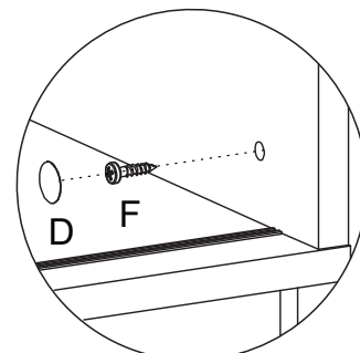
Detalhe 13 Detail/Detalle
