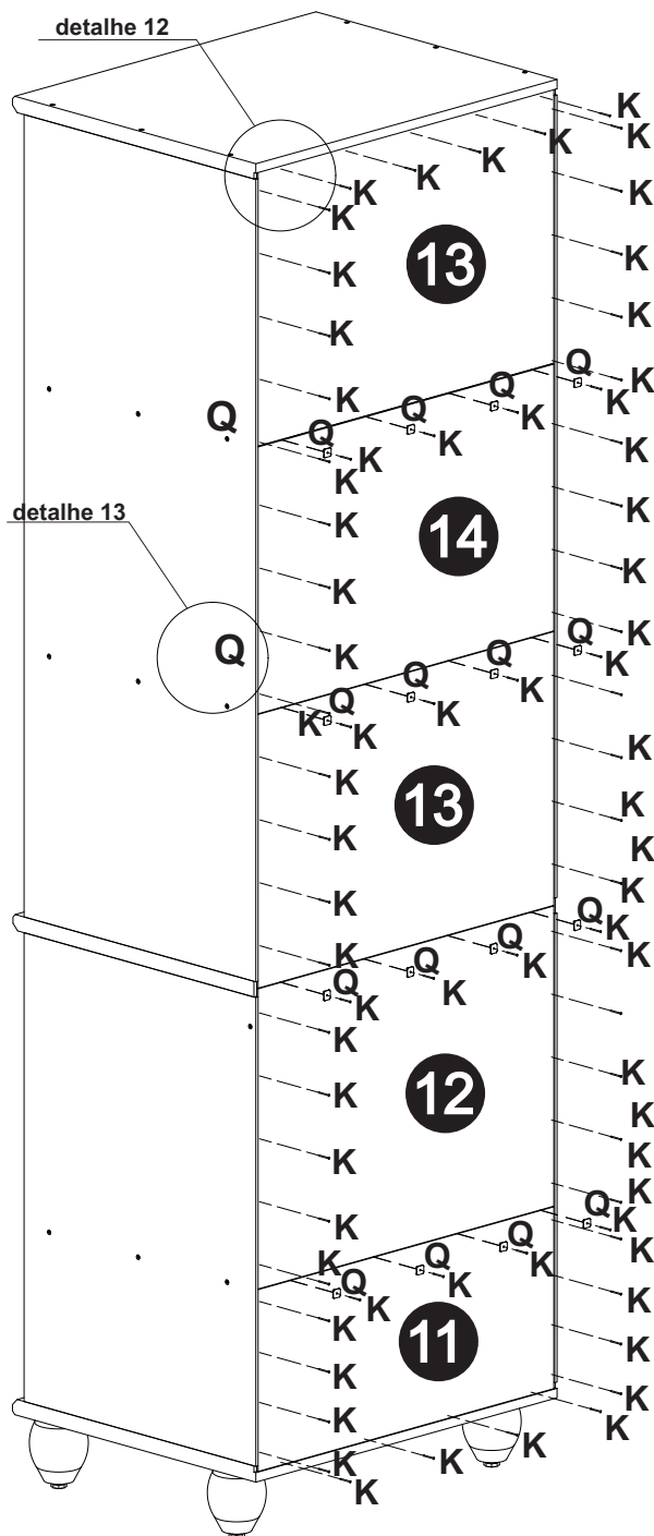
Q- Chapinha Fixa Fundo Cod 0804001 (16x)
