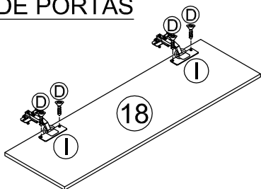
DETALHE DE PORTAS
