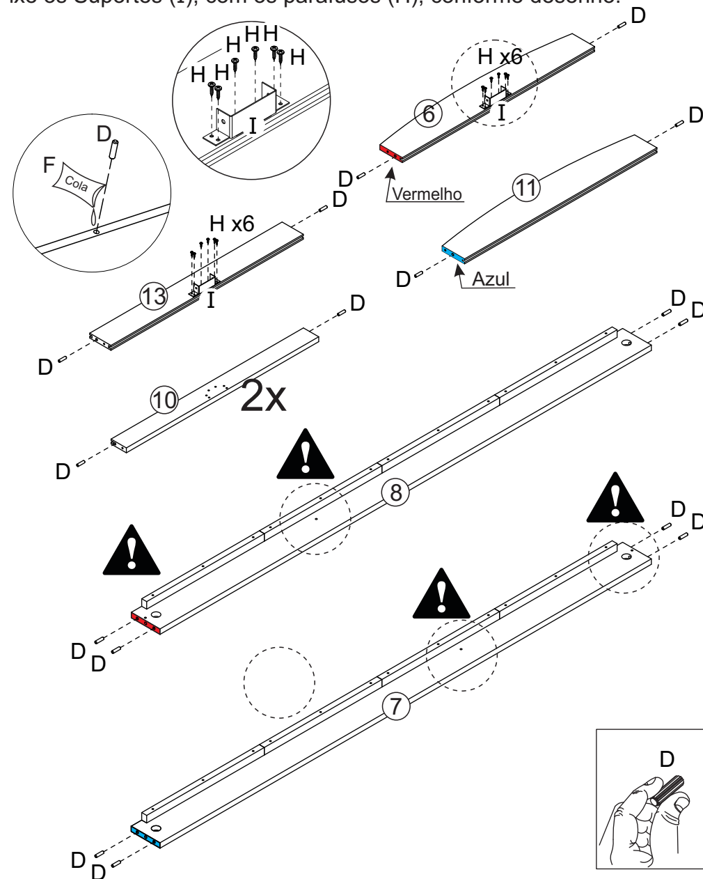
H - Parafuso PH PN 3,5 x 16mm BI Quant. Peças 16
