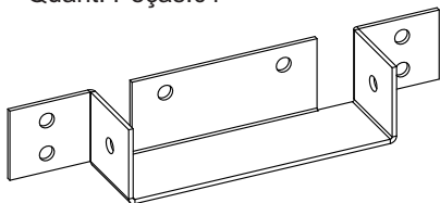
I - Suporte Central Quant. Peças 02
