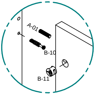
Detalhe B
