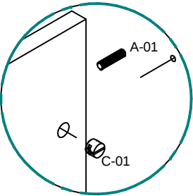
Detalhe C
