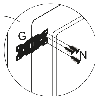
Detalhe 21
