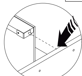
detalhe 05
