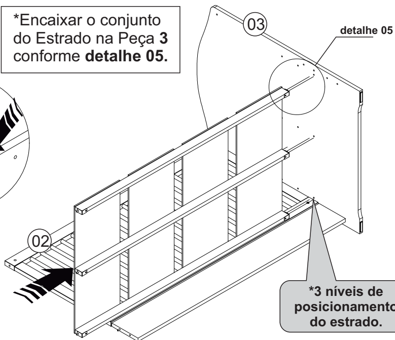
detalhe 05
