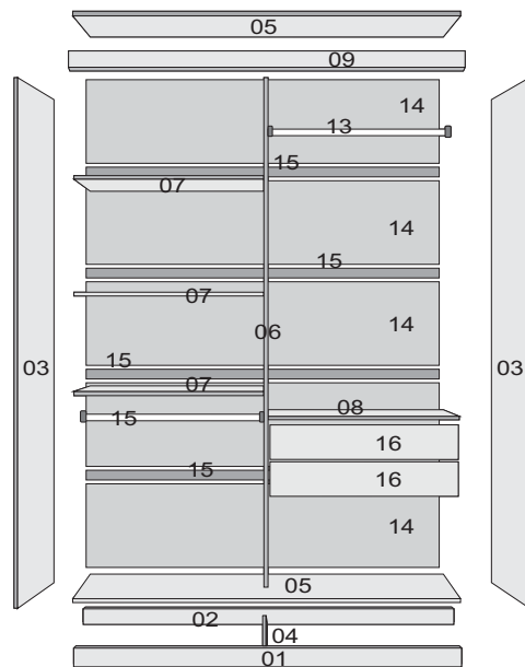
PEÇAS EXPLODIDAS
