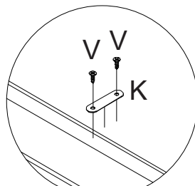
detalhe 17
