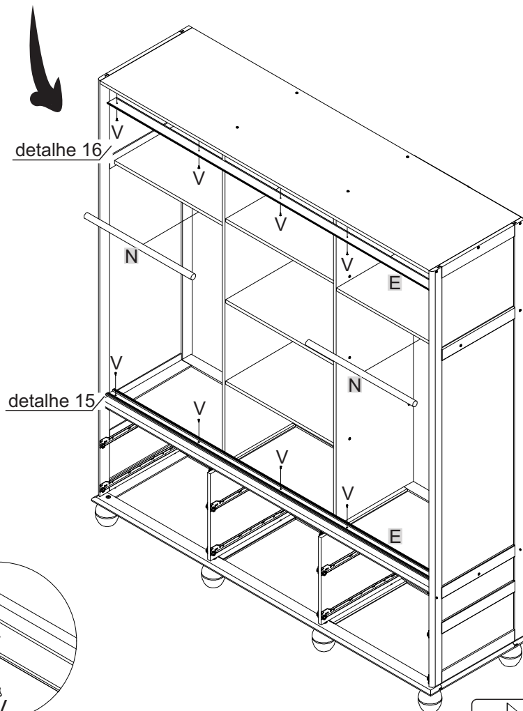
detalhe 16
