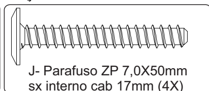
detalhe 7
