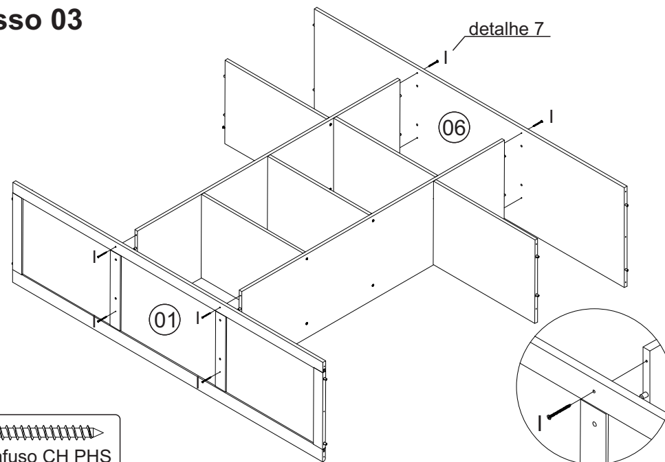
detalhe 7
