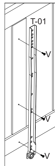
detalhe 11
