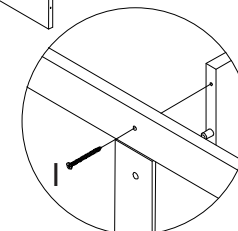
detalhe 7
