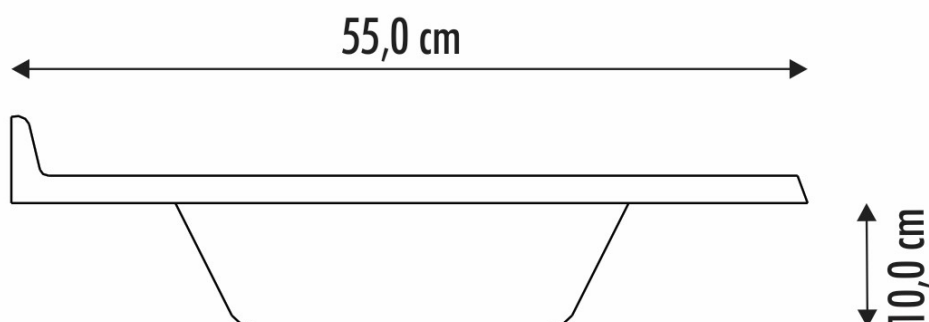
Vista Lateral
