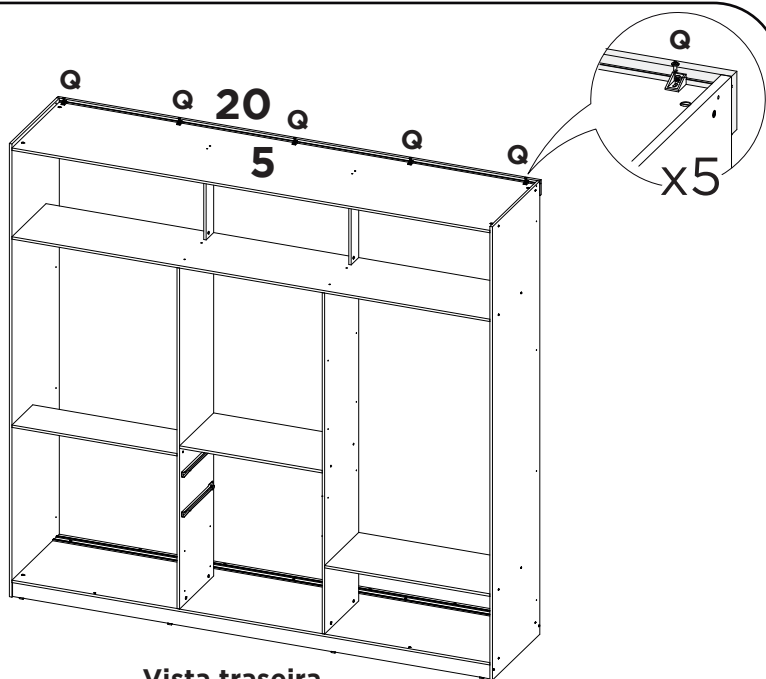
Vista traseira
