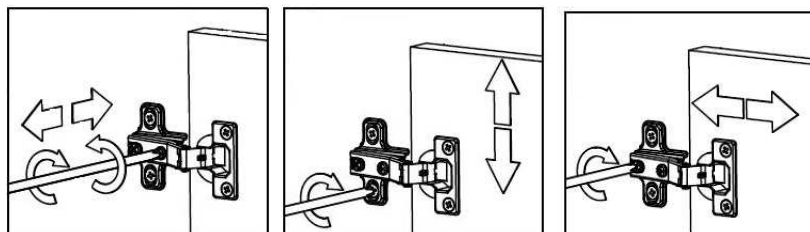
Regulagem das Portas - Door adjustment - Ajuste de la puerta
