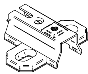
G - Calço (6x)
