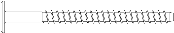
E- Parafuso ø7x90 cab. 17 Quant. Peças: 16
