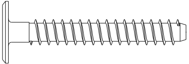
B- Parafuso ø7x50 cab. 17 Quant. Peças: 13
