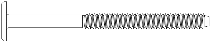
F- Parafuso ø1/4x90 cab. 17 Quant. Peças: 08
