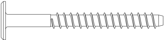
D- Parafuso ø7x70 cab. 17 Quant. Peças: 03
