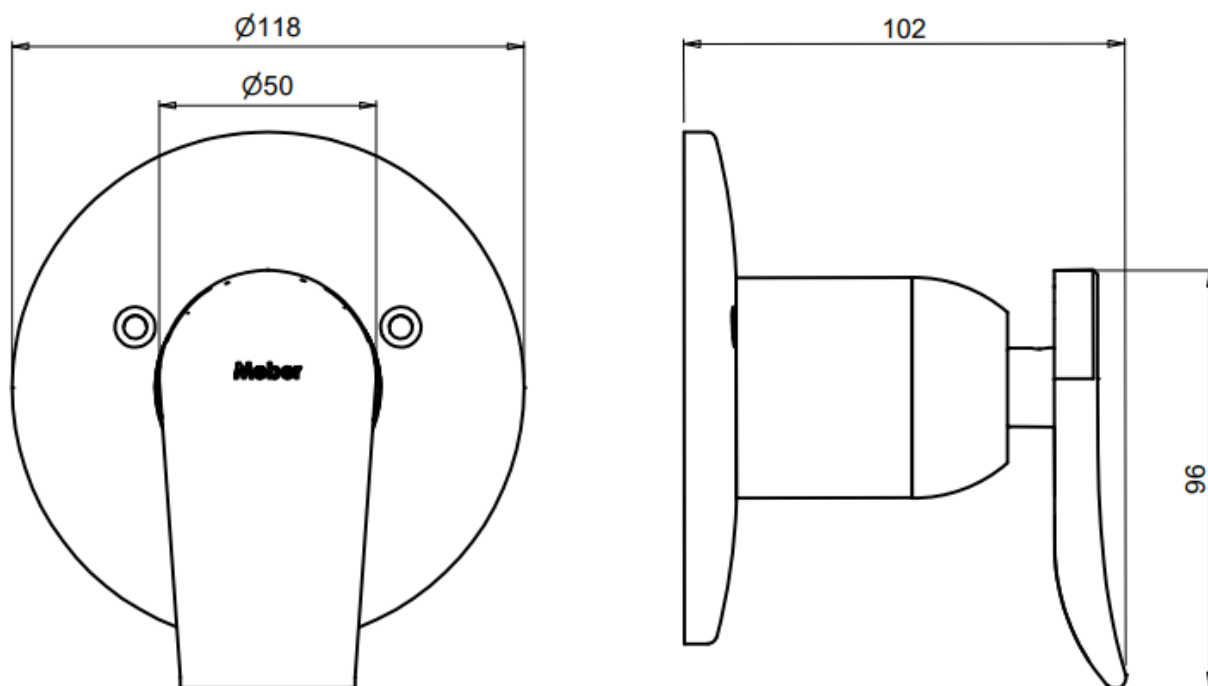
Desenho técnico
