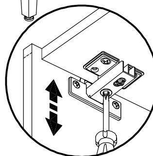
Vertical Adjustment Regulagem Vertical Ajuste Vertical
