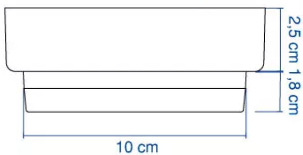
VISTA LATERAL BASE
