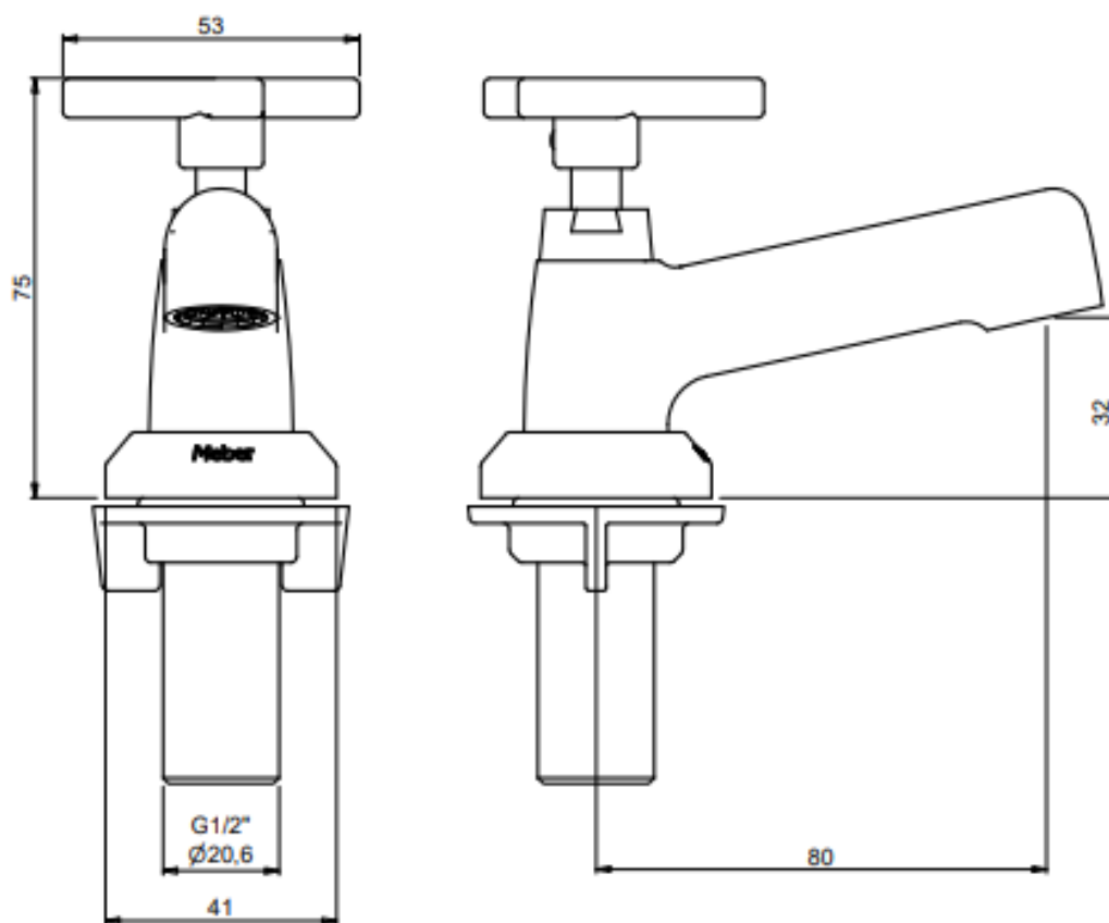
Desenho técnico
