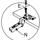
Detalhe 4 detail 4 / detalhe 4
