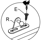
Detalhe 6 detail 6 / detalhe 6
